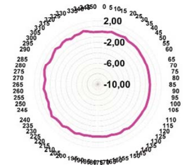
Freq. 900 MHz H-plane (dBi) V-pol
